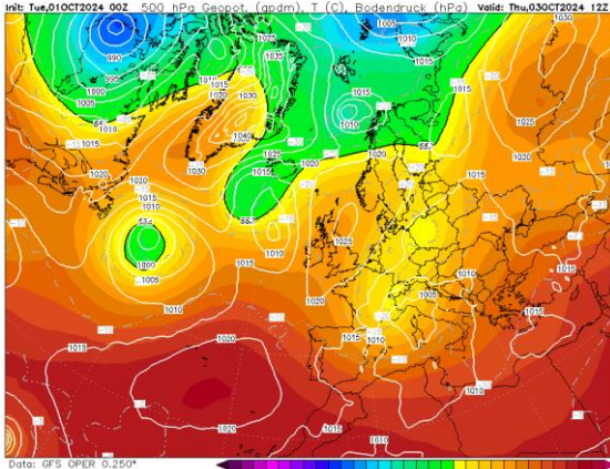
Mapa de 500 hPa 03/10/2024 12 UTC GFS
