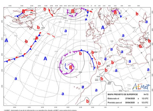
Mapa de superficie 30/04/2025 14:00 h
