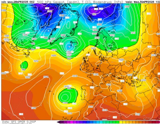
Mapa de 500 hPa 30/04/2025 12 UTC GFS
